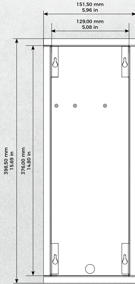
Unterputzgehäuse
