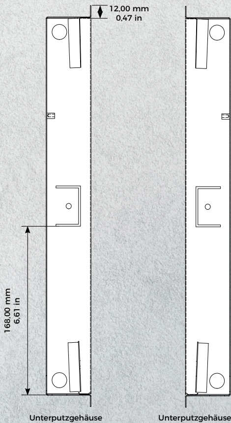
Unterputzgehäuse
