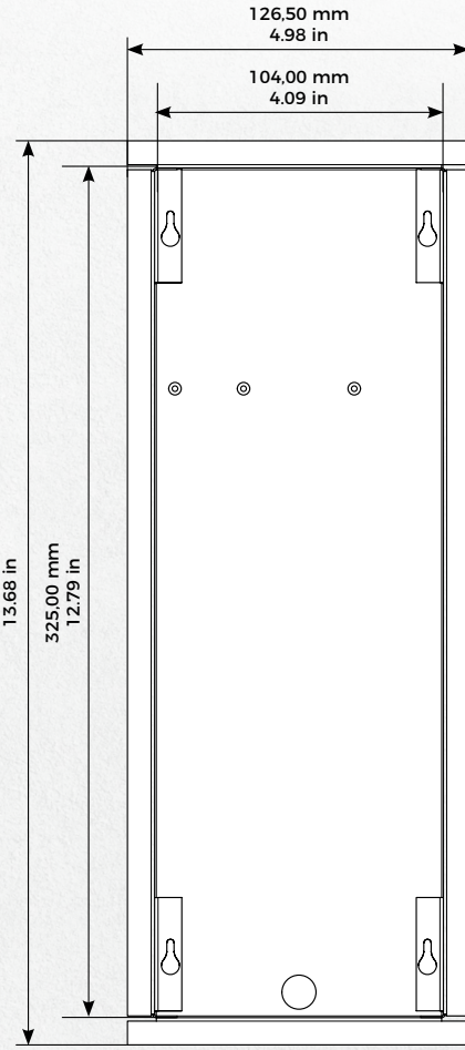
Unterputzgehäuse
