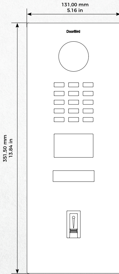
Frontblende
