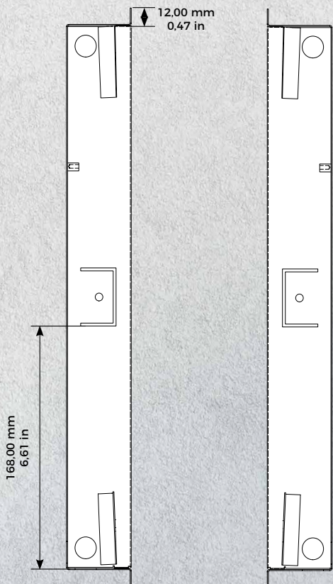
Unterputzgehäuse
