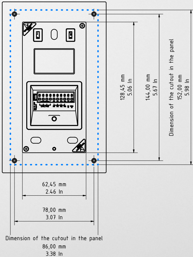
Rückseite
