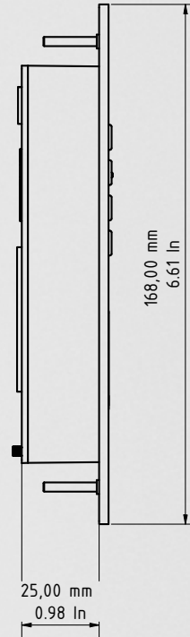
Seite
