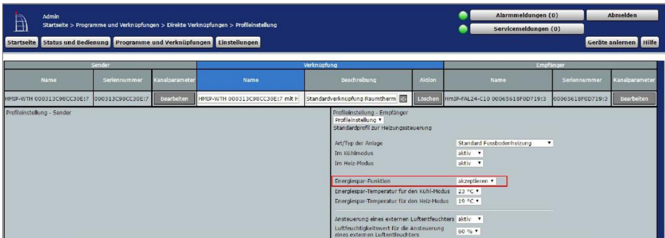
Abbildung 241: Verknüpfungparameter zwischen Wandthermostat und Fußbodenheizungsaktor
