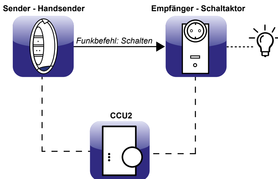
Abbildung 40: Kommunikation bei einer direkten Geräteverknüpfung mit Zentrale
