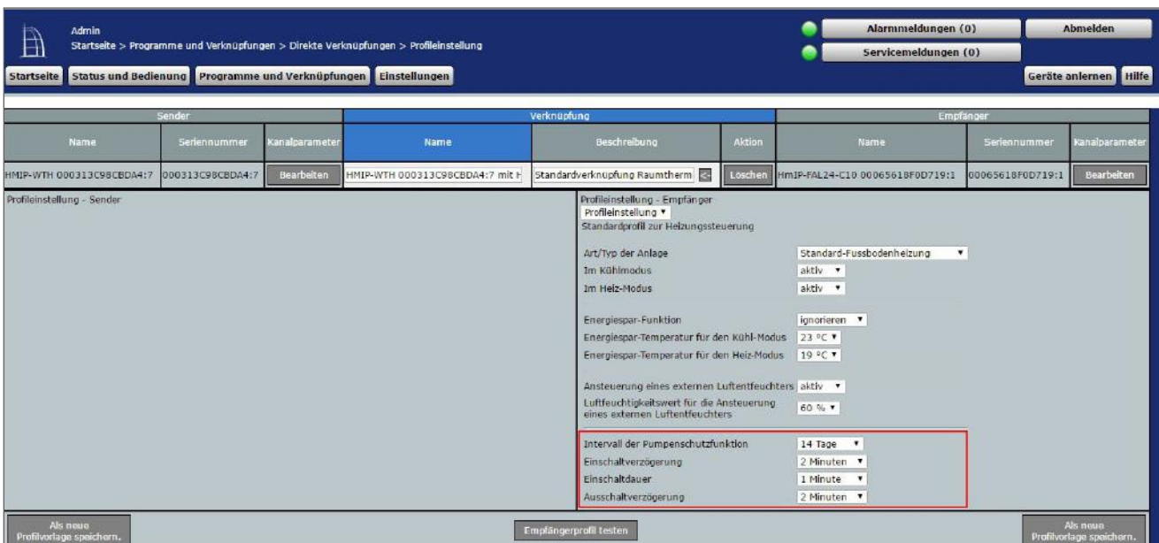
Abbildung 242: Verknüpfungparameter zwischen Wandthermostat Kanal 1 (Pumpe) und Fußbodenheizungsaktor
