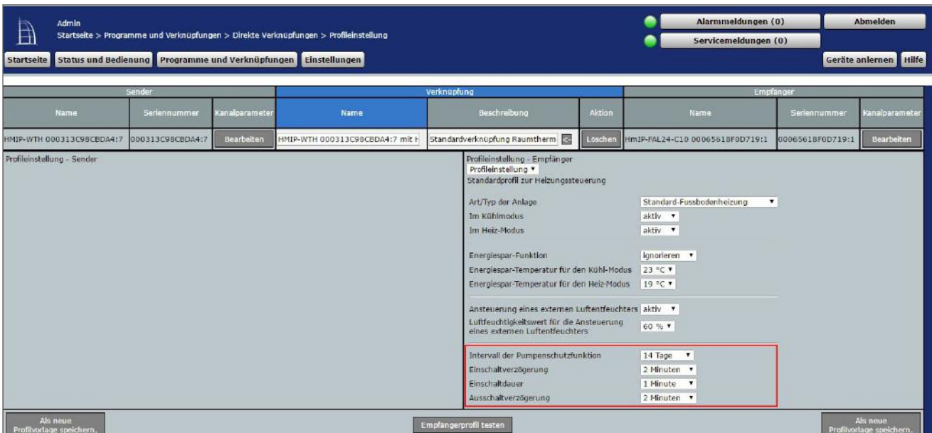
Abbildung 251: Verknüpfungsparameter zwischen Wandthermostat Kanal 1 (Pumpe) und Fußbodenheizungsaktor
