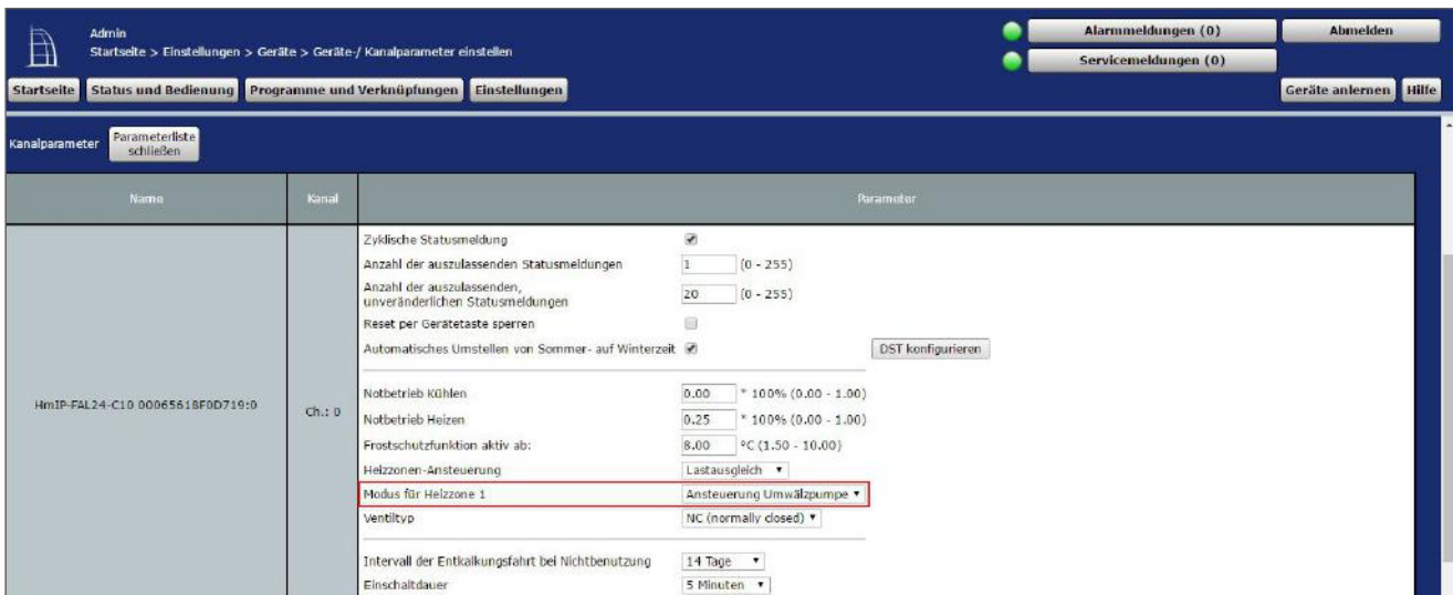
Abbildung 253: Konfiguration Fußbodenheizungsaktor
