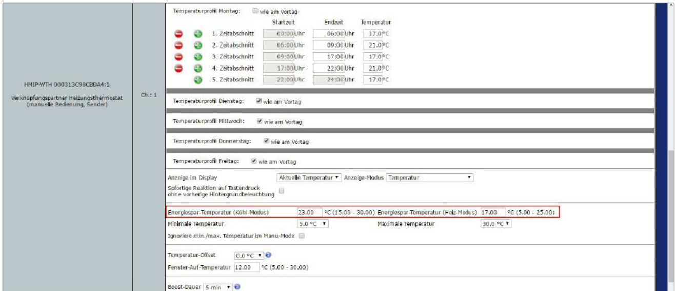
Abbildung 254: Konfiguration Fußbodenheizungsaktor
