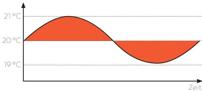
Standard Thermostat mit Zweipunktregelung
