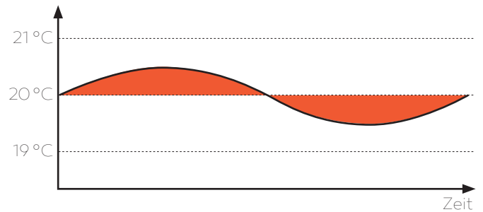
Welltherm Thermostat mit selbstlernender Regelung
