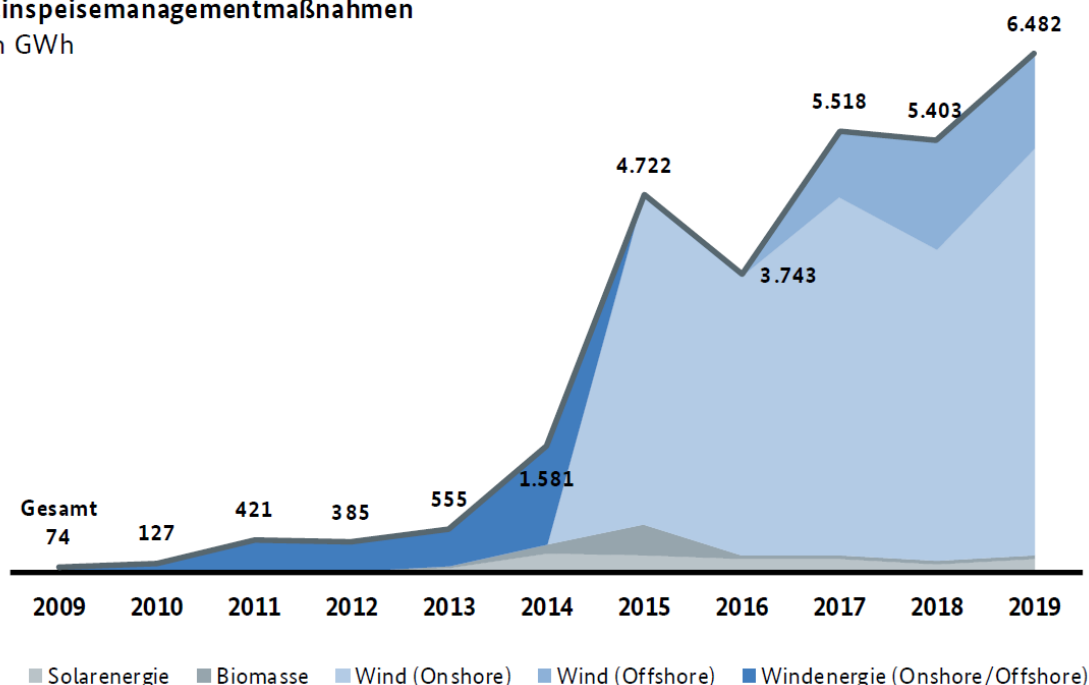
Abbildung 22: Abgeregelter elektrische Energie [BNA]
