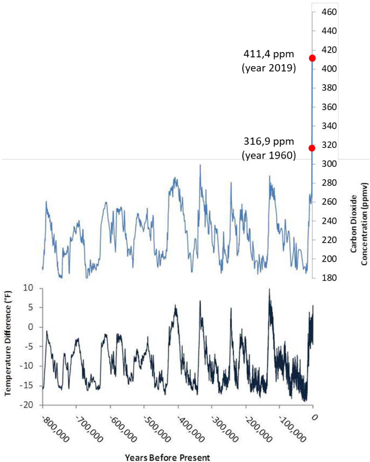
Abbildung 37: Schätzungen der atmosphärischen CO 2 -Konzentration und der Temperatur in der Antarktis auf Basis von Eisbohrkernen [EPA] mit zwei neueren Messwerten des Mauna Loa Observatory [ https://www.esrl.noaa.gov/gmd/ccgg/trends/data.html ]
