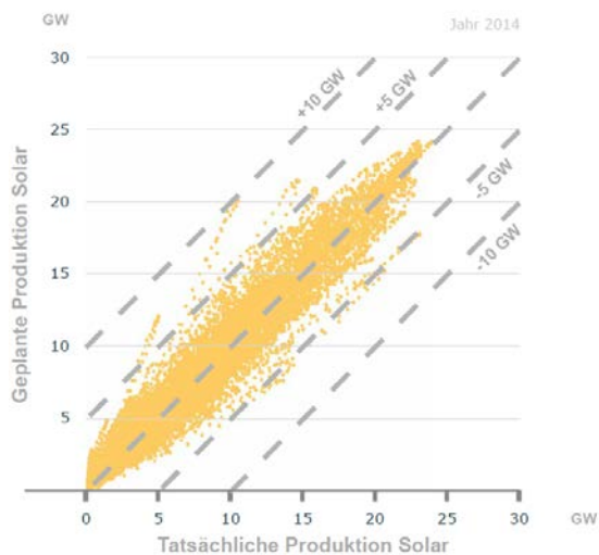
Abbildung 23: Stündliche tatsächliche und geplante Stromproduktion im Jahr 2014 [ISE4]
