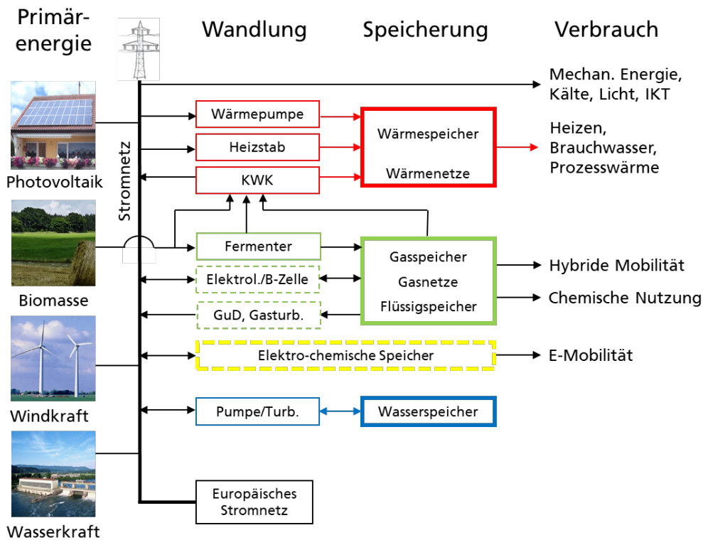
Abbildung 59: Vereinfachte schematische Darstellung eines Erneuerbaren Energiesystems mit den wichtigsten stromnetzgebundenen Bausteinen der Kategorien Gewinnung, Wandlung, Speicherung und Verbrauch
